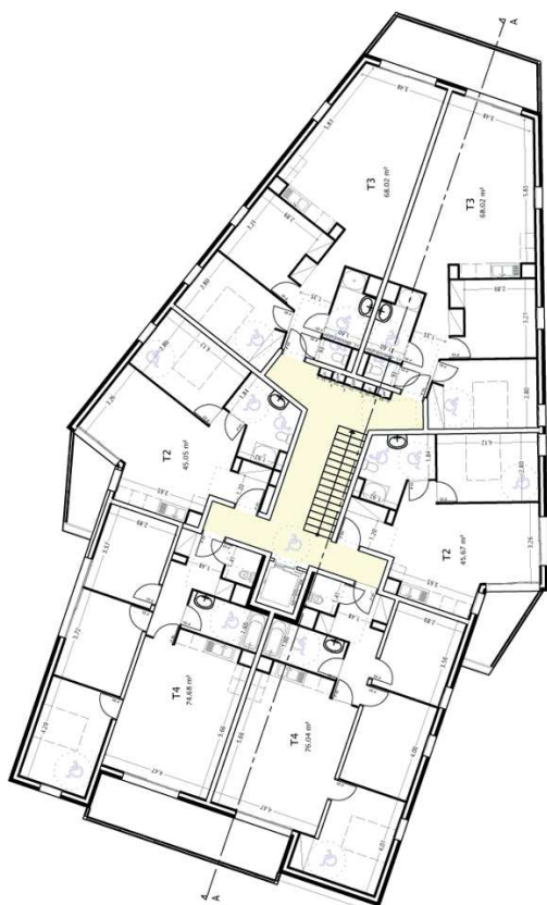
ETAGE COURANT
